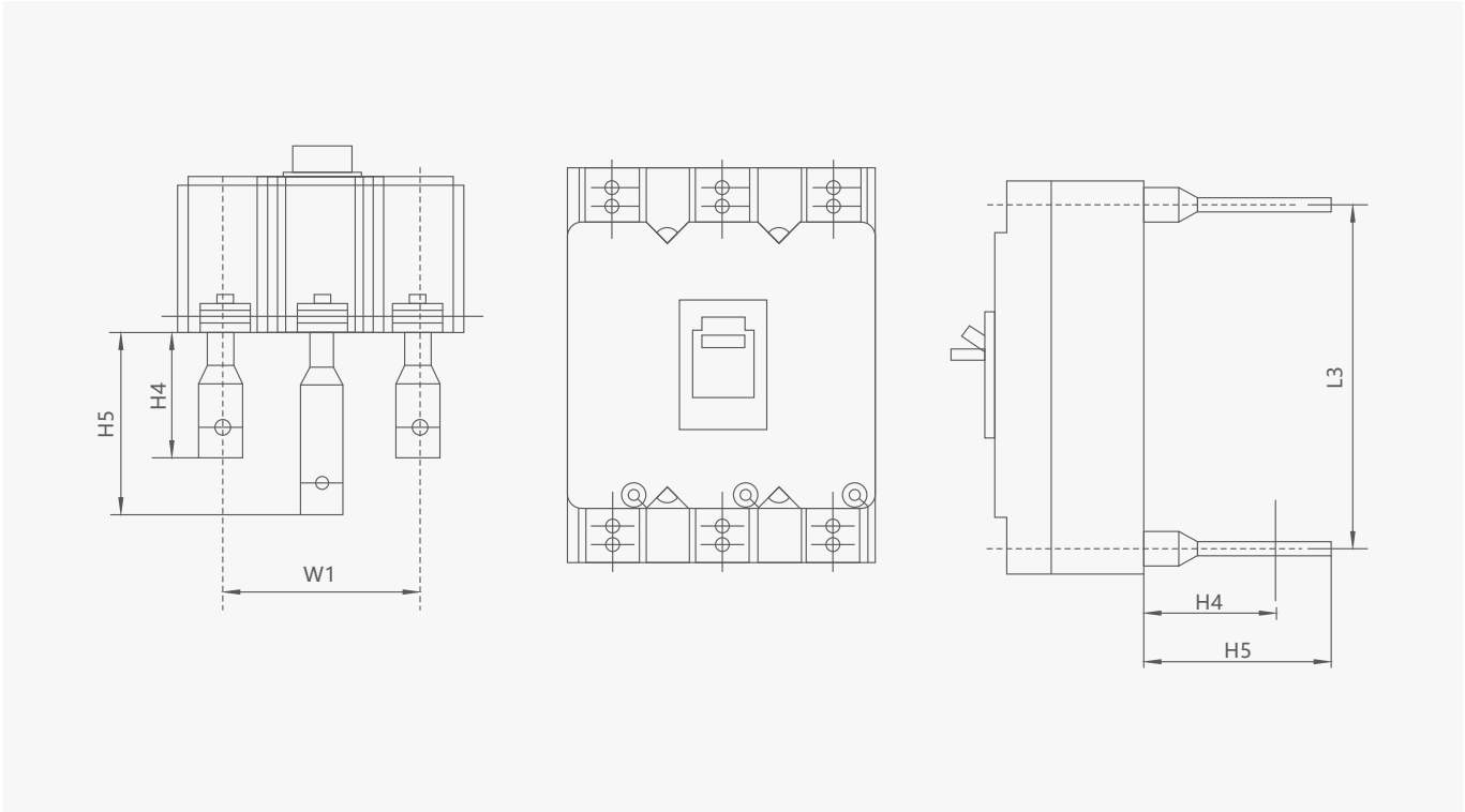
板后接线
