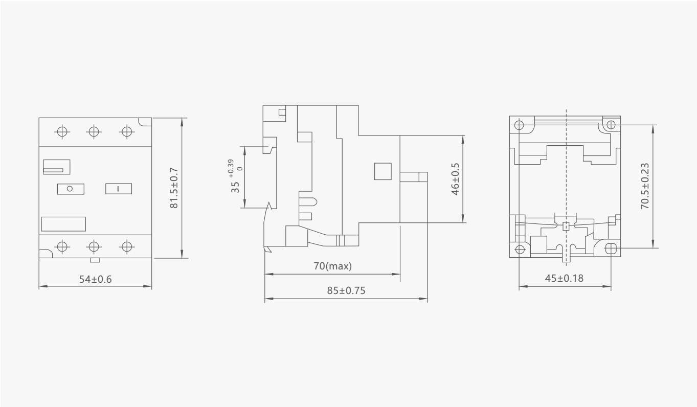
DZ108-20外形及安装尺寸
