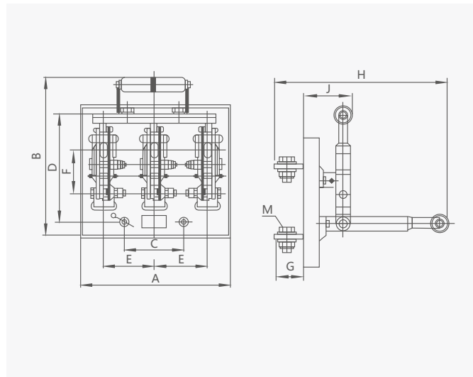
HS12-100~400、HS12B-100~400接线图(尺寸见E表)
