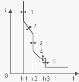
电子式脱扣器保护特性曲线
